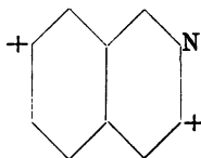
δ Disulfosäure.
